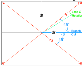
fig.3. for 45^\circ - 45^\circ eq.9 case: leptons
